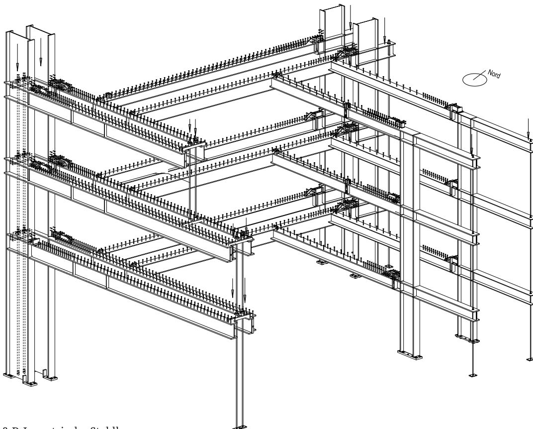
3-D-Isometrie des Stahlbaus
